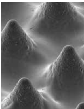
Typische RoundTop-Rasterpunkte
